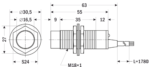
AR-LM18-3008NC NPN
