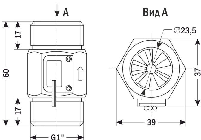
Рис. 2 – Размеры прибора
